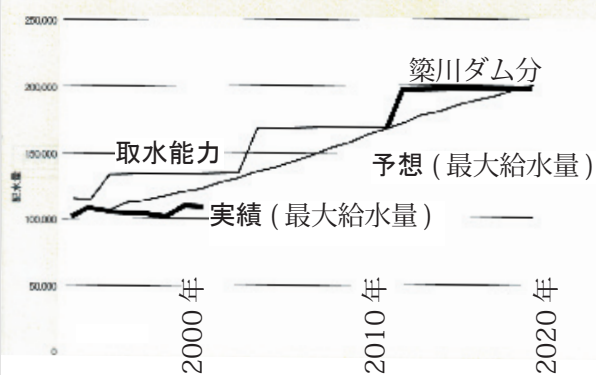
盛岡市の水道用水計画図
