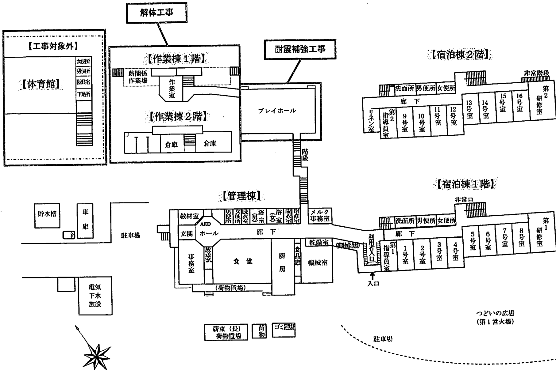
施設平面図
