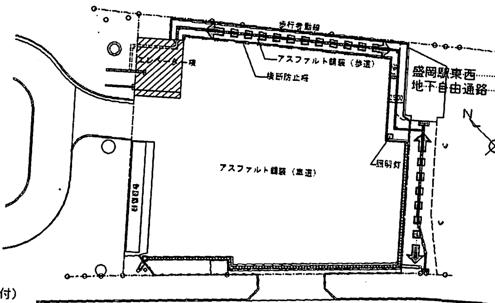
バス乗場平面図
